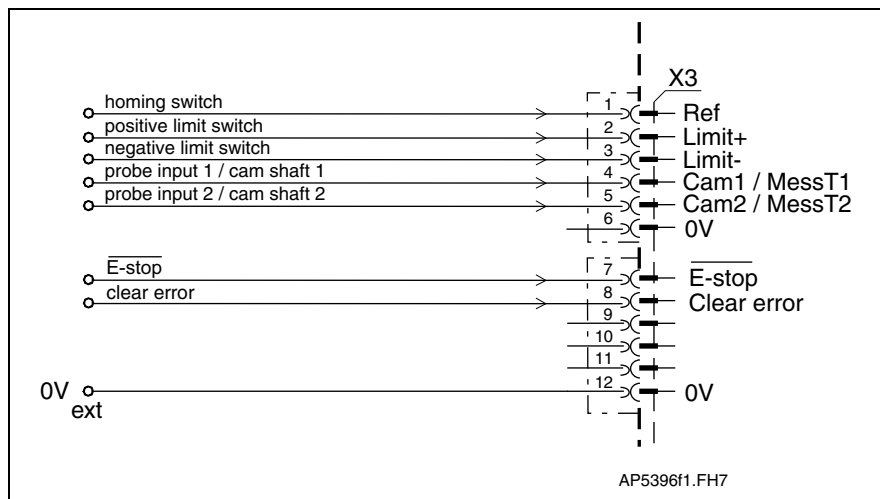
Fig. 5-38: Digital inputs
