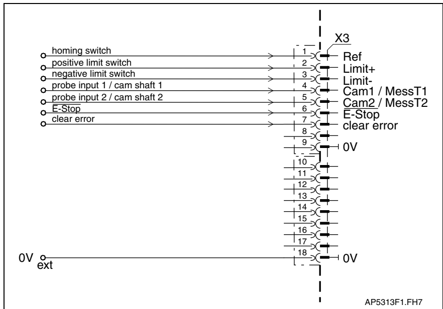
Fig. 4-66: Digital inputs
