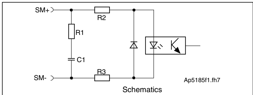
R1: 121R R2: 121R R3: 121R C1: 1 nF Fig. 4-170: Differential input circuit
