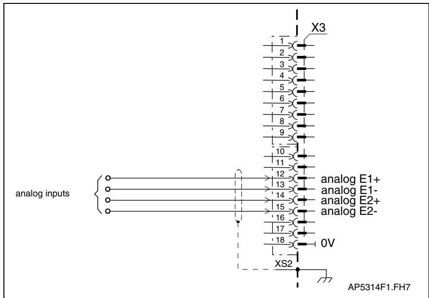
Fig. 4-76: Analog inputs
