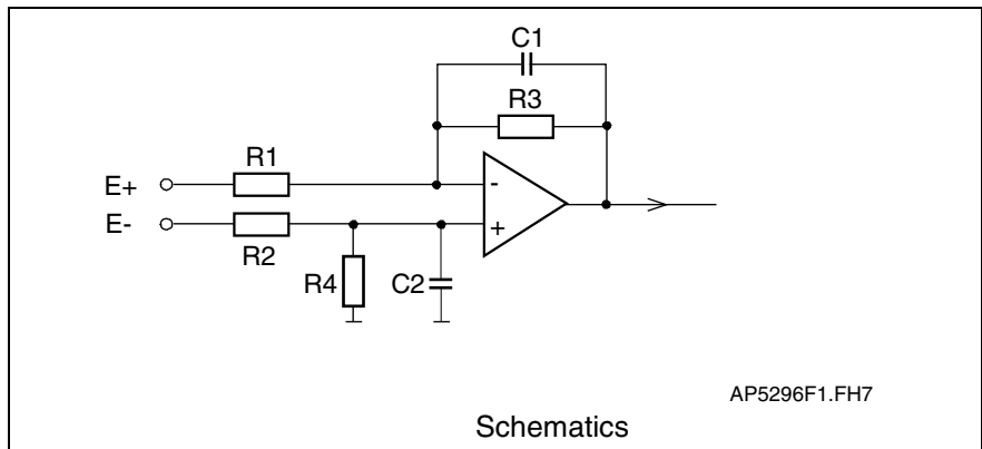
Fig. 4-76: Analog inputs
